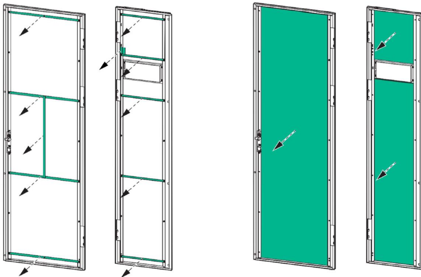
Рисунок 15-2. ИБП мощностью 500-600 кВА
