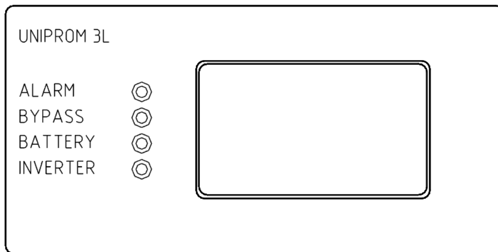
Рисунок 6-1. Пользовательский интерфейс
