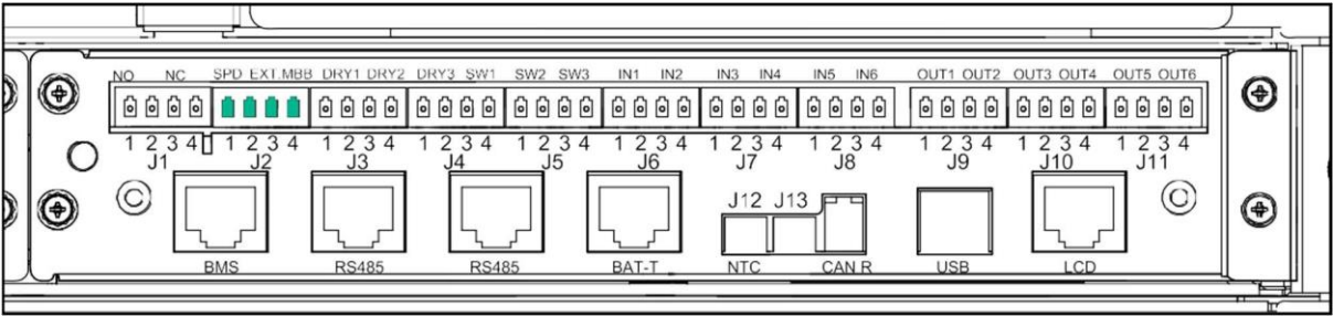
Рисунок 17-13. Сервисный байпас
