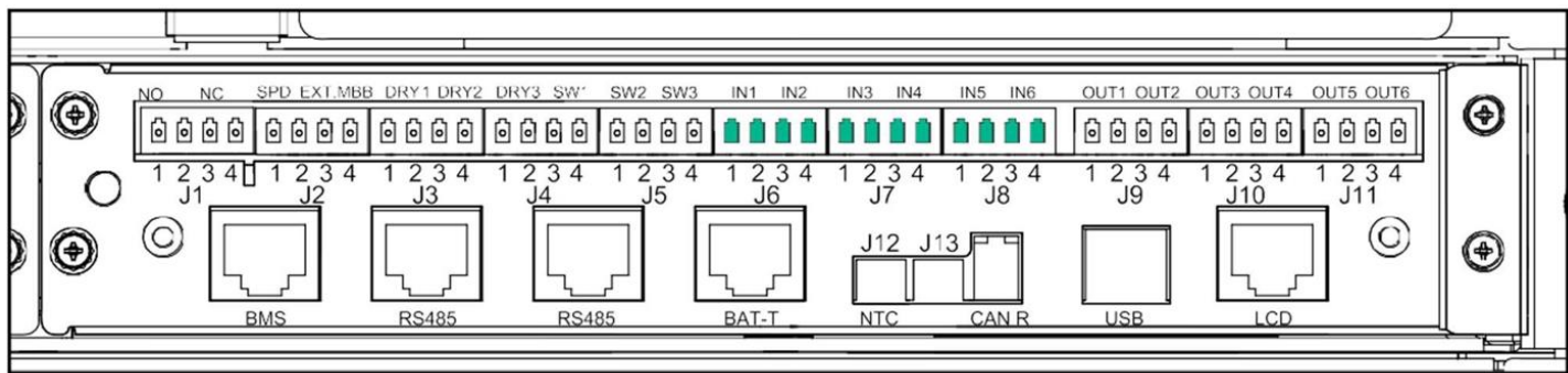
Рисунок 17-15. Входные сигналы
