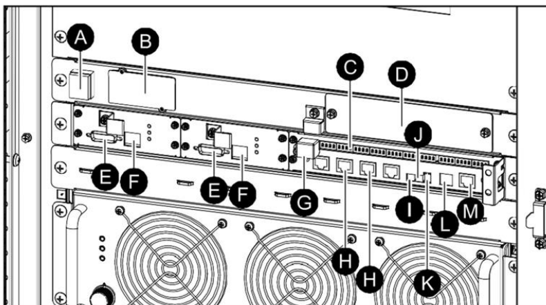
Рисунок 17-7. Блок управления
