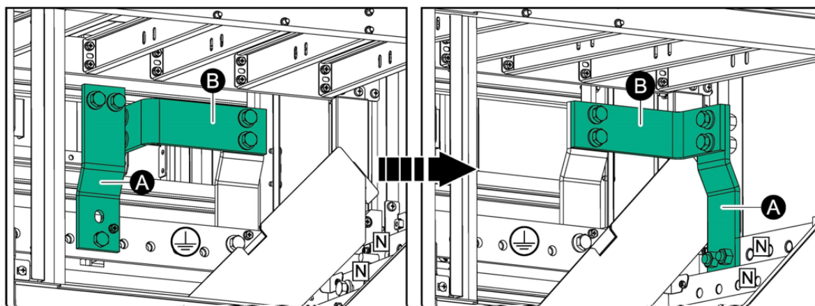
Рисунок 17-5. Система TNC
