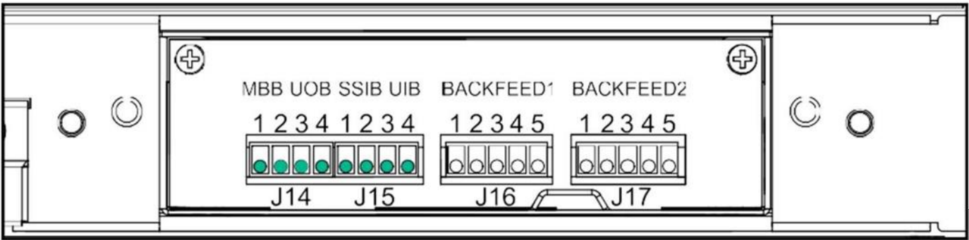
Рисунок 17-11. Сигнальные входы
