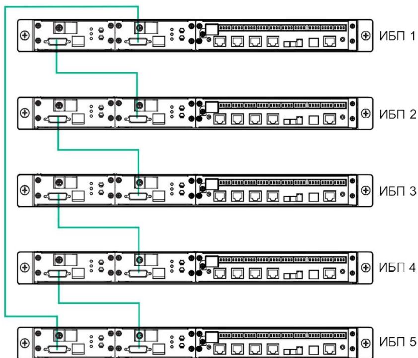
Рисунок 17-17. Параллельная работа ИБП
