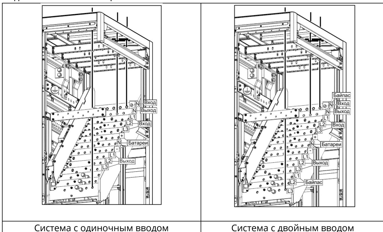
Рисунок 17-6. Подключение кабелей
