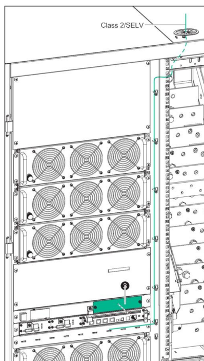
Рисунок 17-9. Точки подключения
